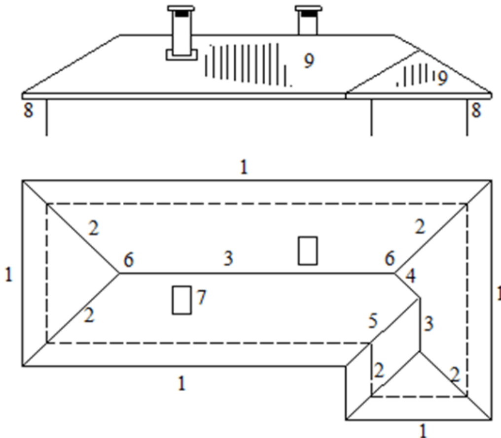
Obrázok č. 1 – Plán strechy s názvami jej prvkov
